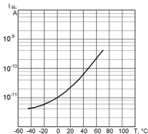
Типовая зависимость входного тока от температуры среды
