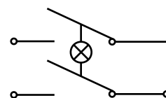
Схема работы переключателя
